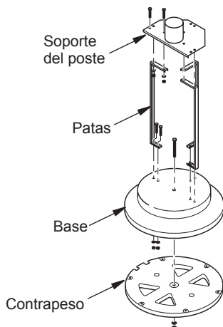
Figura 1 - Ensamblaje de la base
