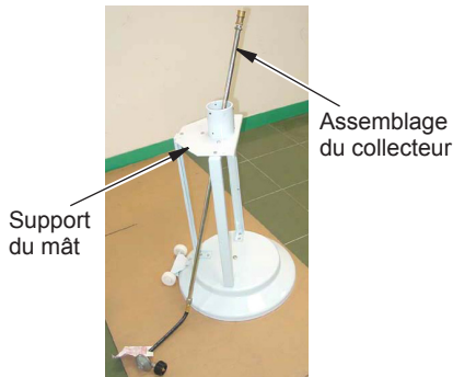
Figure 2 - Installation de l'assemblage du collecteur
