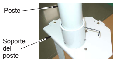
Figura 3 - Poste al soporte del poste
