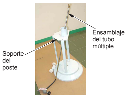
Figura 2 - Instalación del ensamblaje del tubo múltiple
