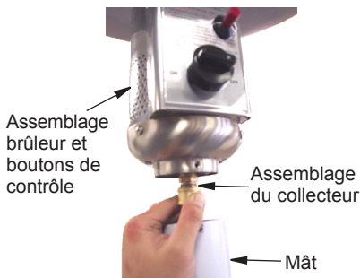
Figure 5 - Raccordement de l'assemblage du collecteur à l'assemblage brûleur et boutons de contrôle
