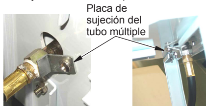
Figura 7 - Fijación de la placa de sujeción del tubo múltiple al soporte del poste
