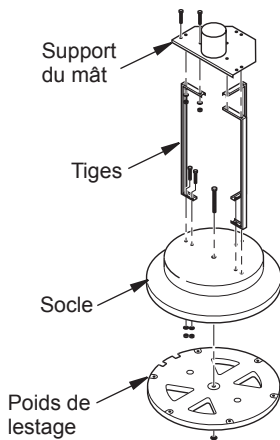
Figure 1 - Assemblage du socle
