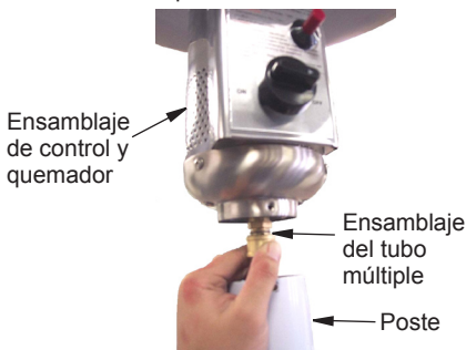
Figura 5 - Conexión del ensamblaje del tubo múltiple al ensamblaje de control y quemador
